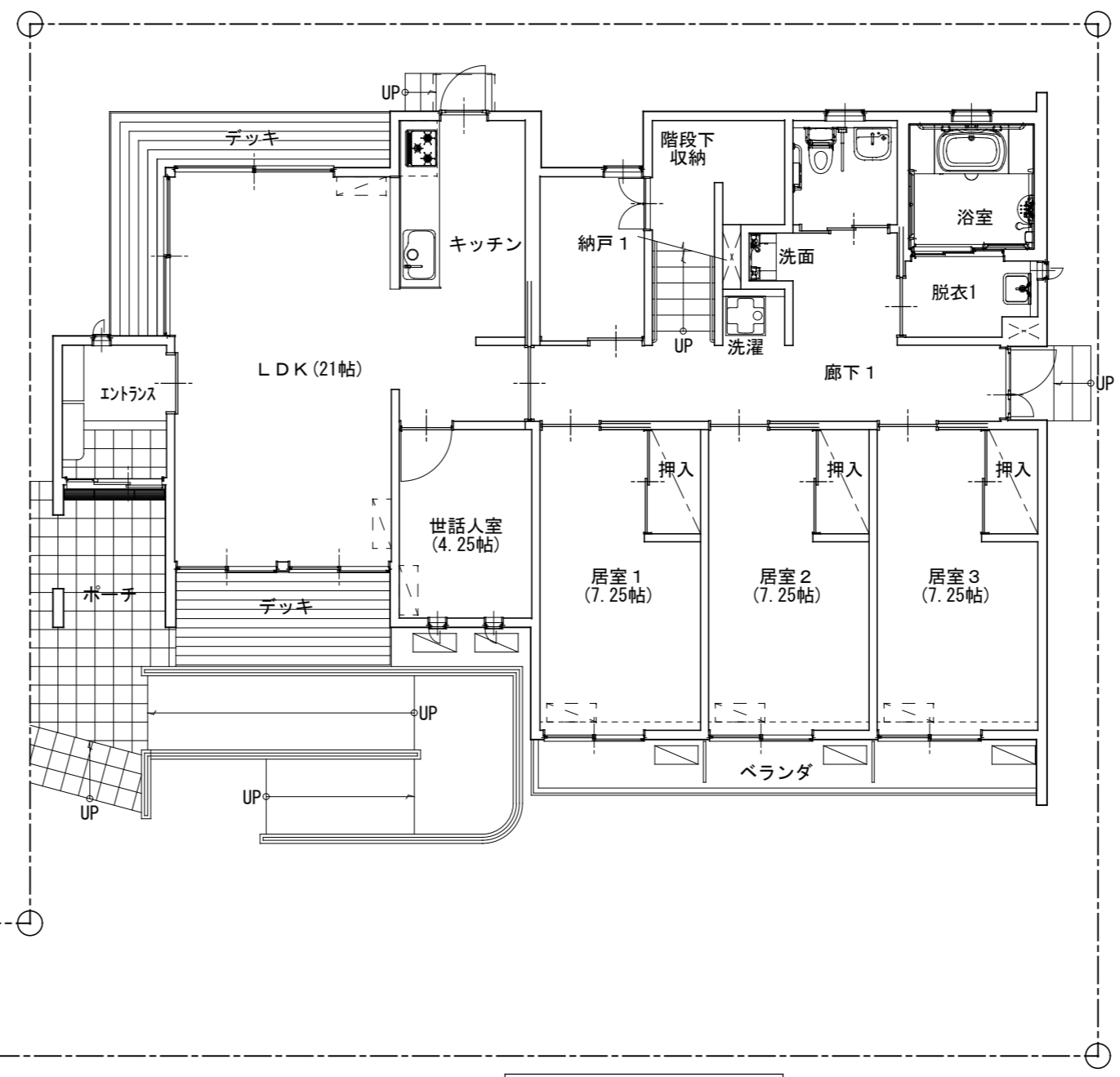
1階平面図
