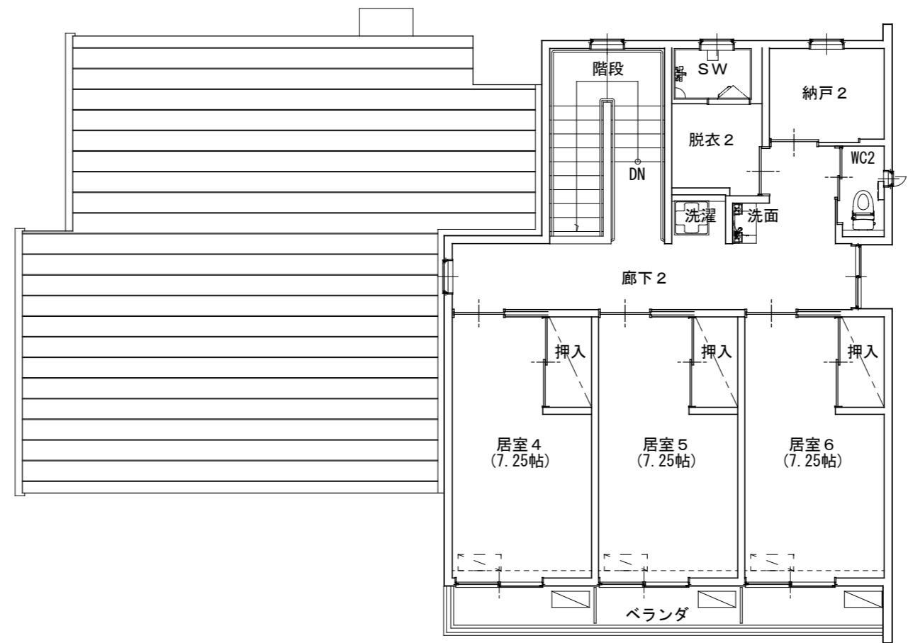
2階平面図
